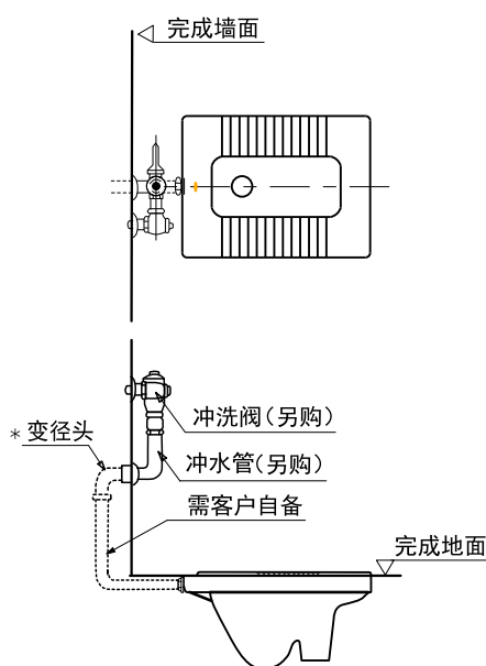
蹲便器配套手压式冲洗阀的安装示意图 (暗装冲水管)
