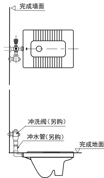
蹲便器配套脚踏式冲洗阀的安装示意图 (明装冲水管)
