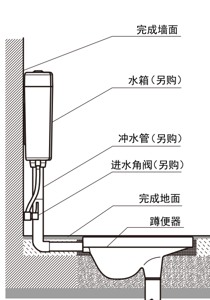
蹲便器配套水箱的安装示意图 (明装冲水管)
